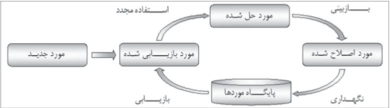
شکل ۱- مراحل مختلف کار در فرایند استدلال مبتنی بر مورد
