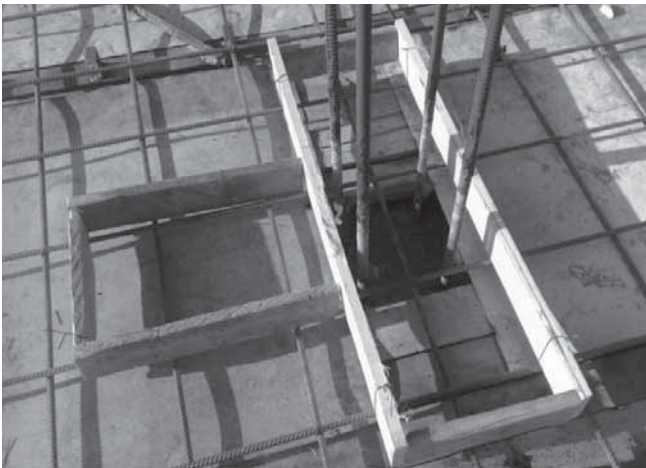
شکل ۴-۵ قالب بندی چوبی
